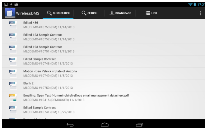
Android
